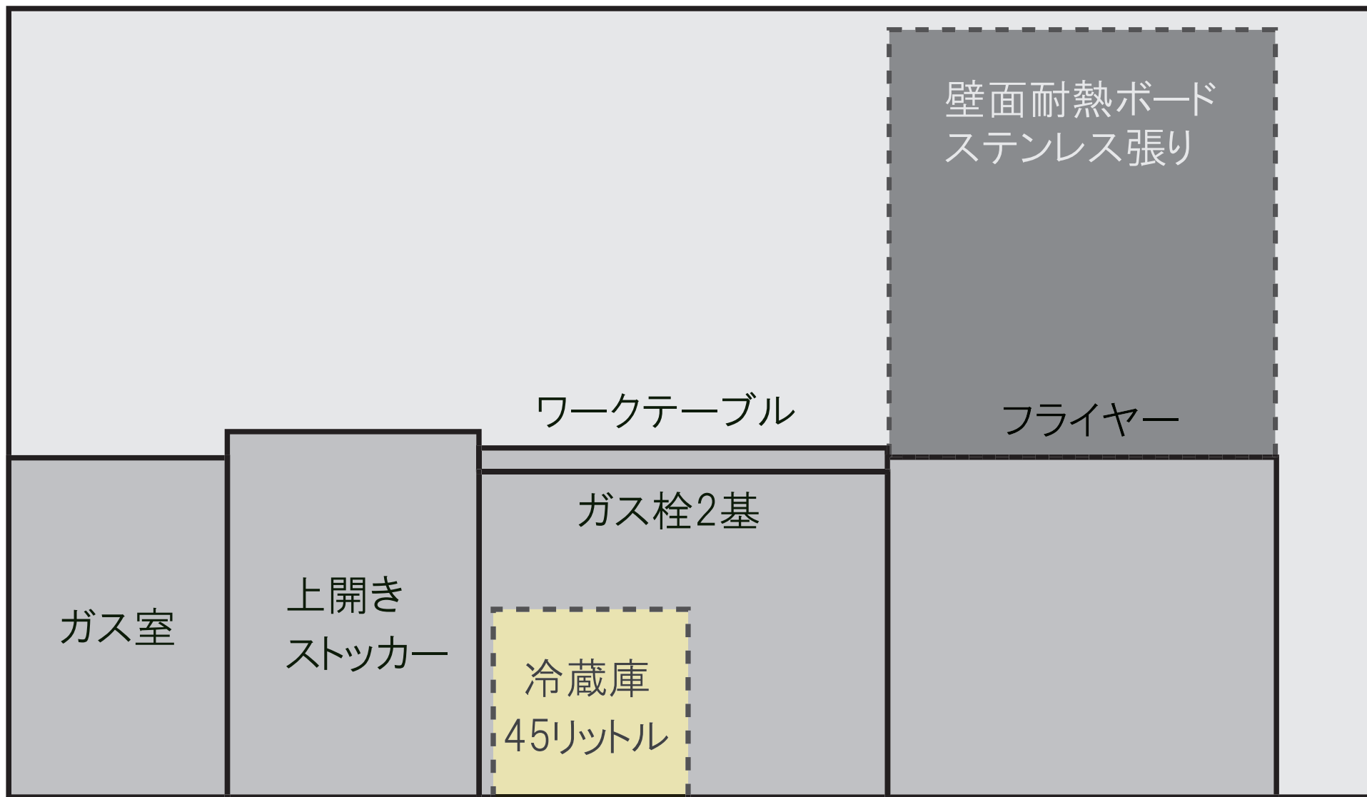
「立面図(右)」
